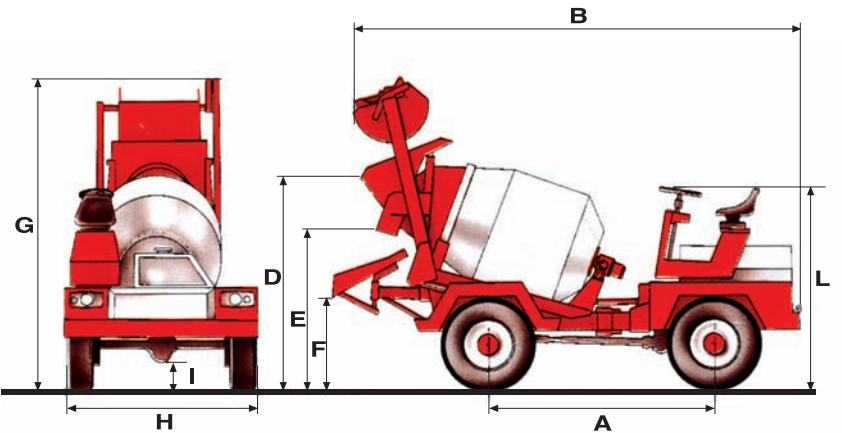
DIMENSIONI - DIMENSION - DIMENSIONS - DIMENSIONAS
